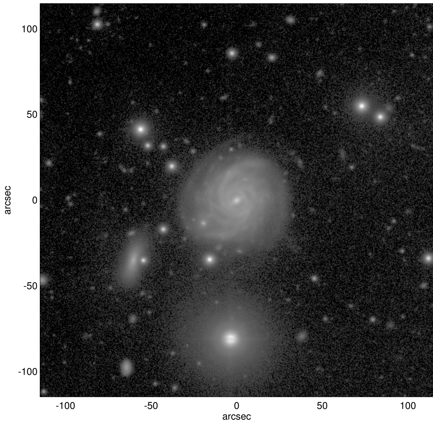
UGC02705
