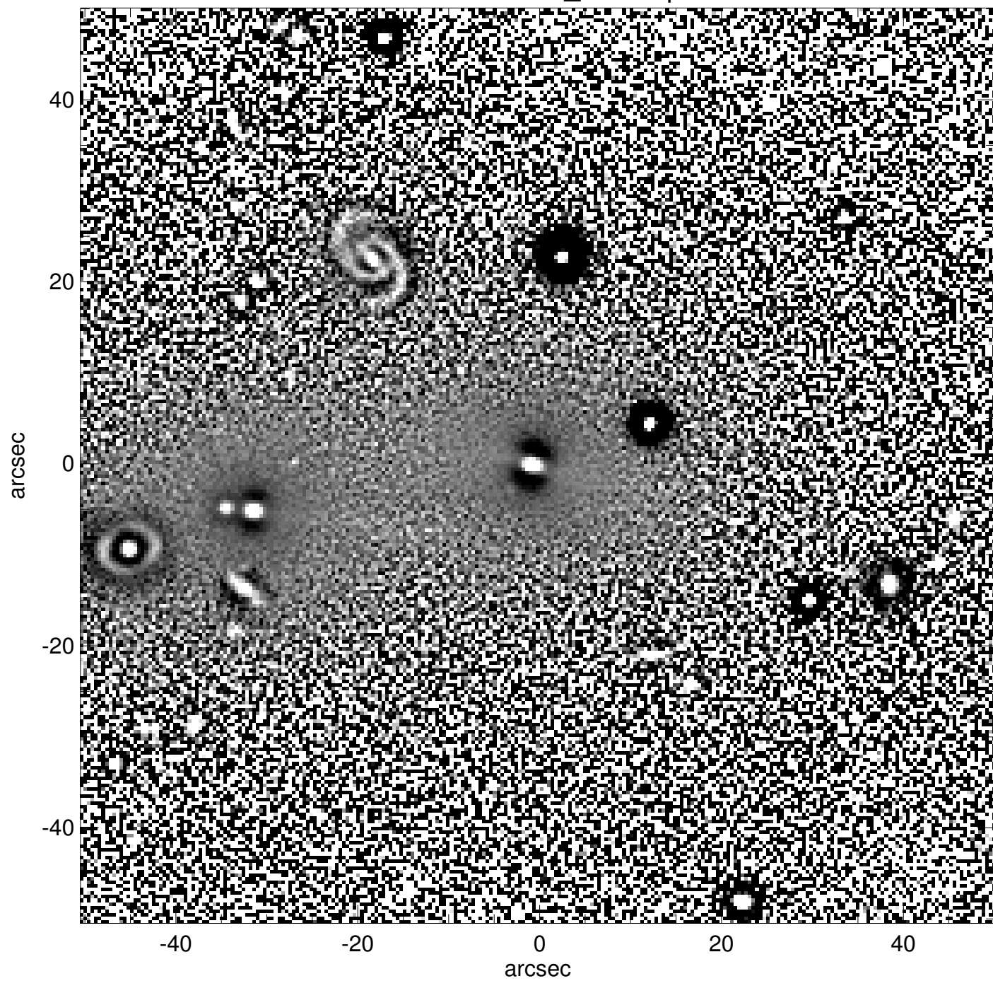
PGC0012694_unsharp
