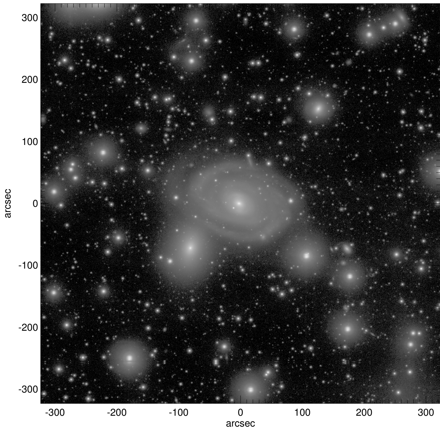
NGC6962
