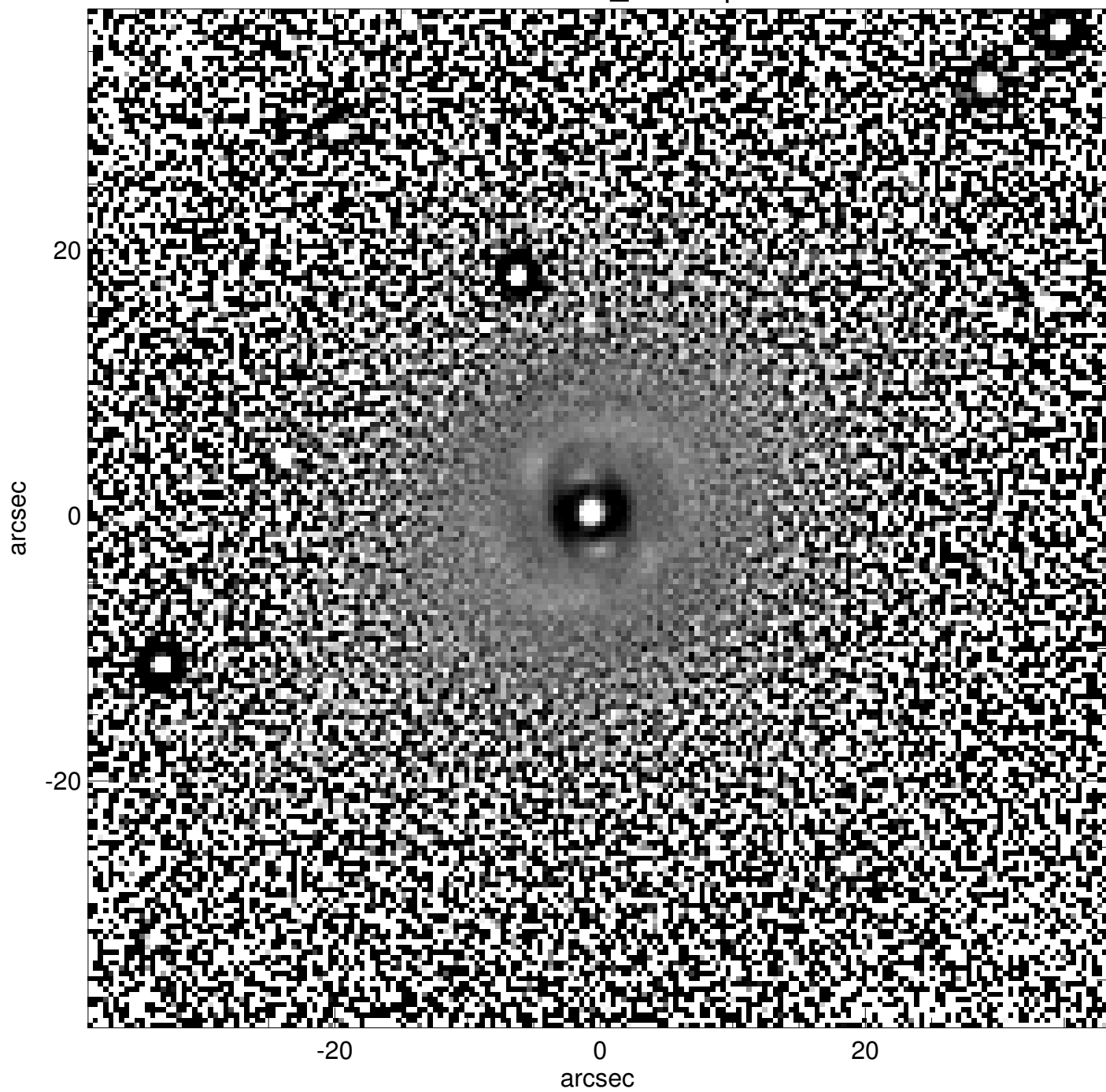
UGC00750_unsharp
