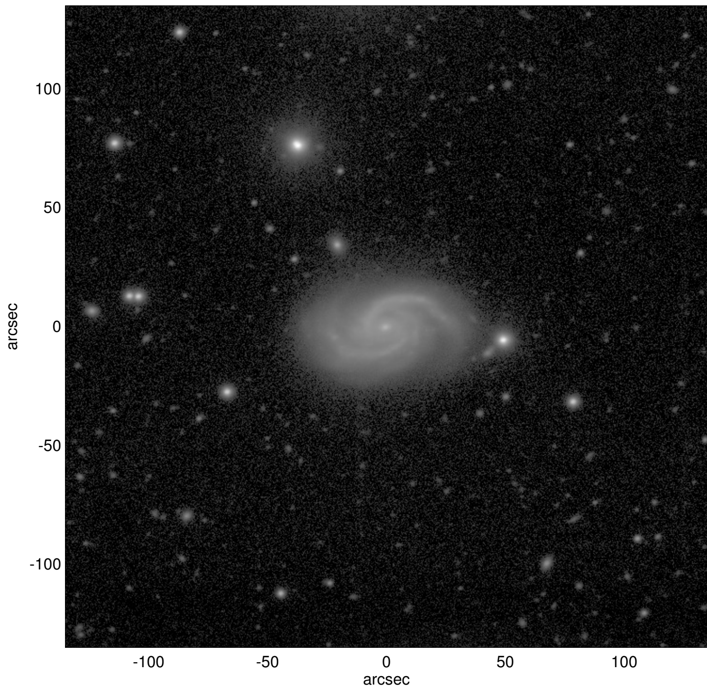
UGC02418
