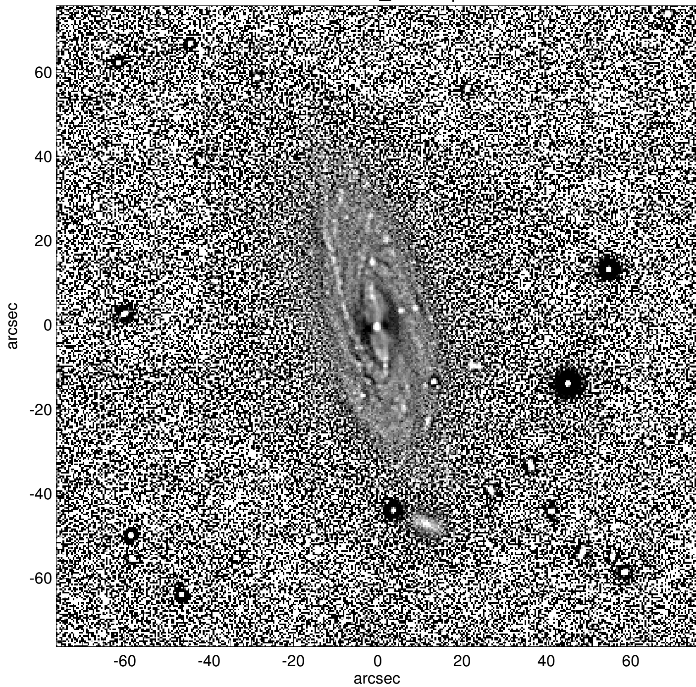
NGC1072_unsharp
