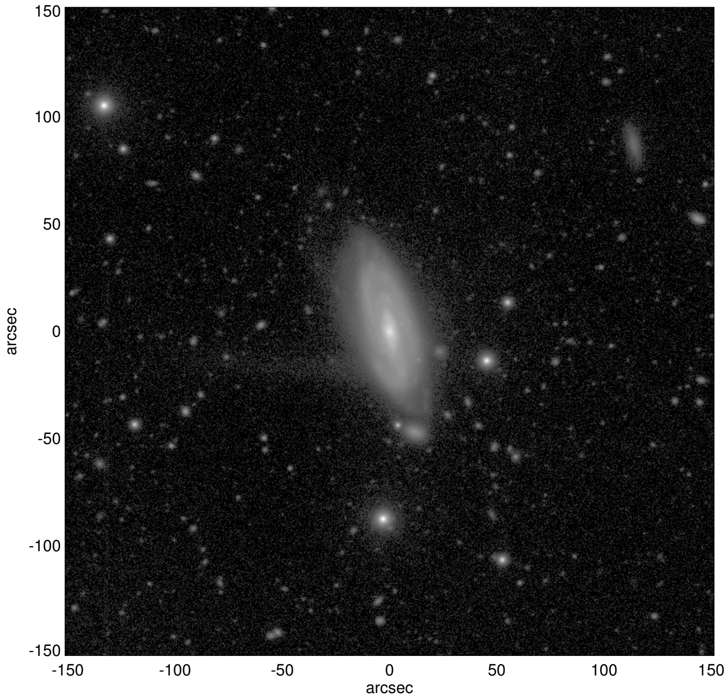
NGC1072
