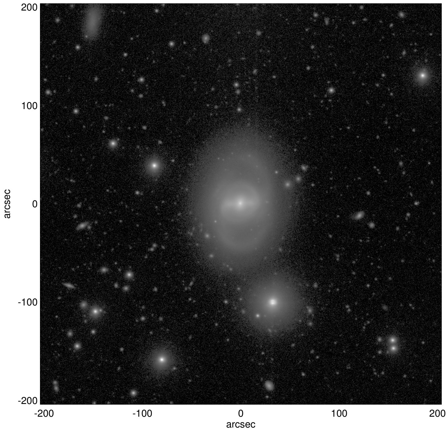
NGC0570
