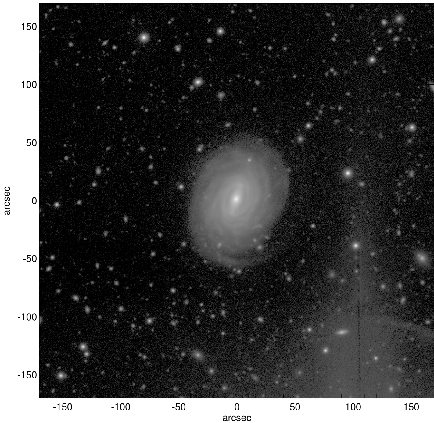
UGC02585
