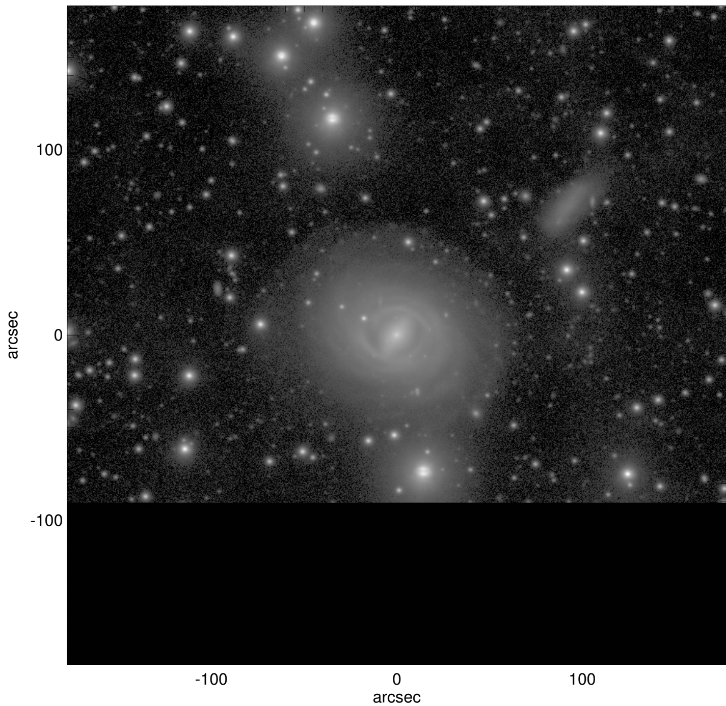
UGC11649
