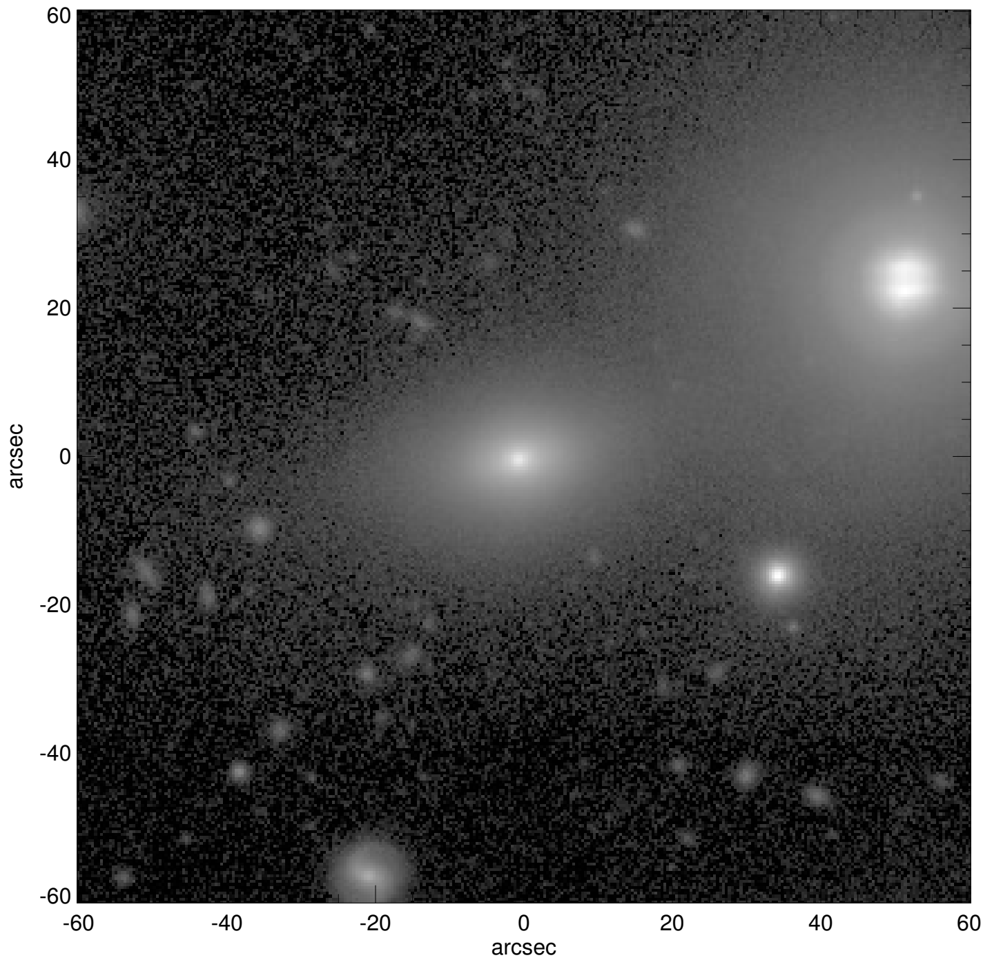
PGC1149561
