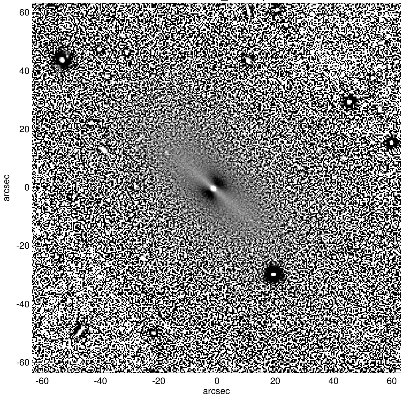
UGC00928_unsharp
