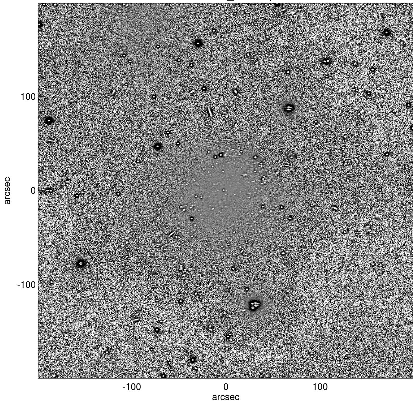
NGC0428_unsharp
