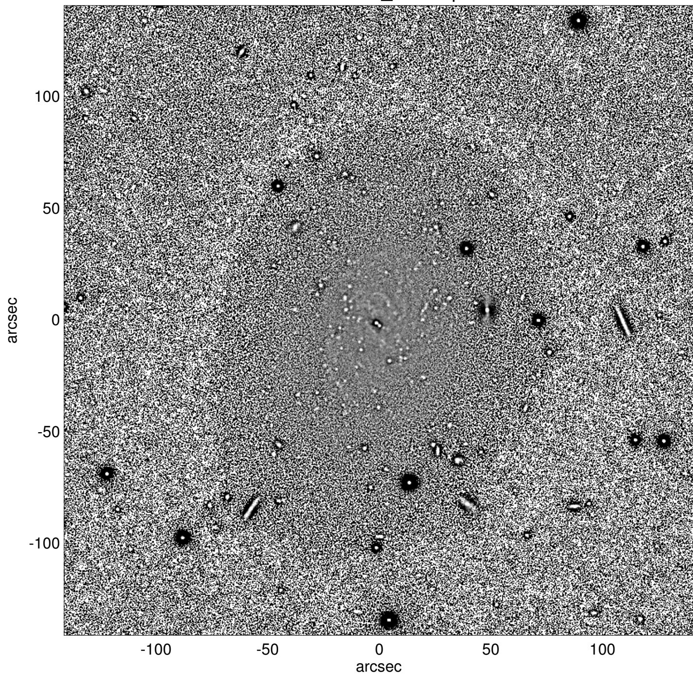
NGC0941_unsharp
