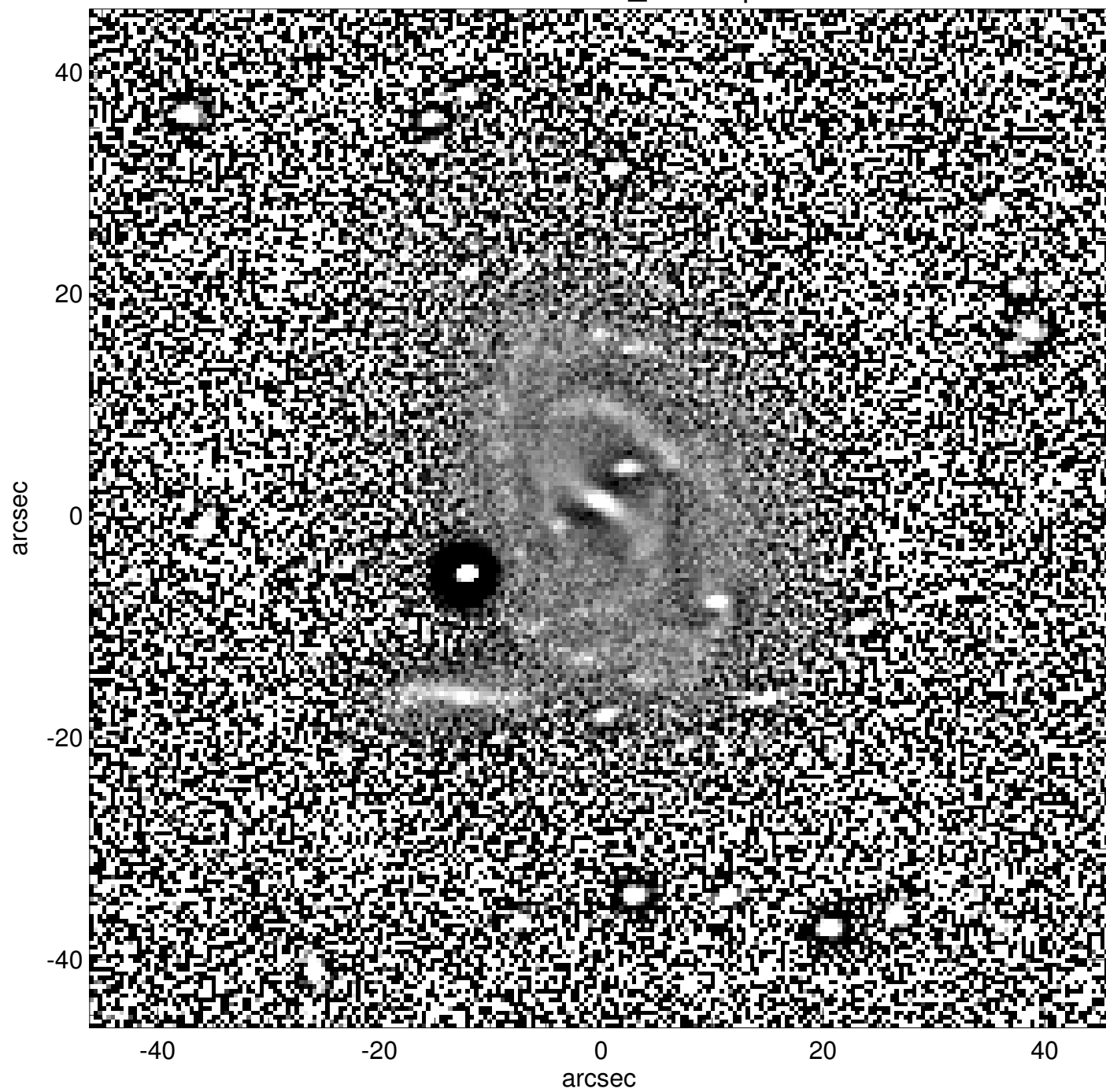
PGC0002484_unsharp
