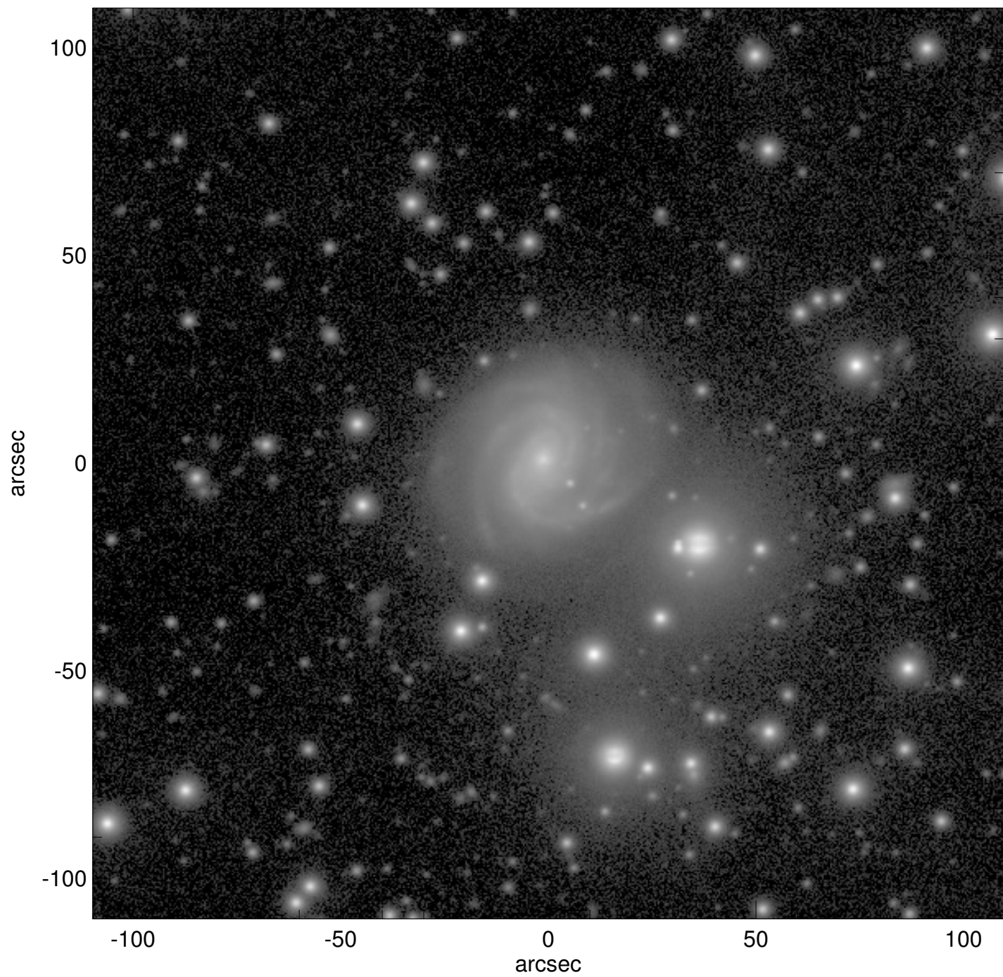
PGC0065616
