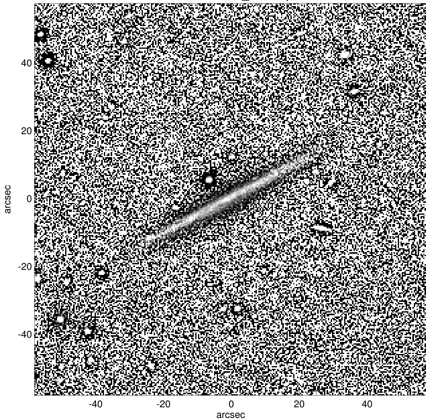
PGC0090504_unsharp
