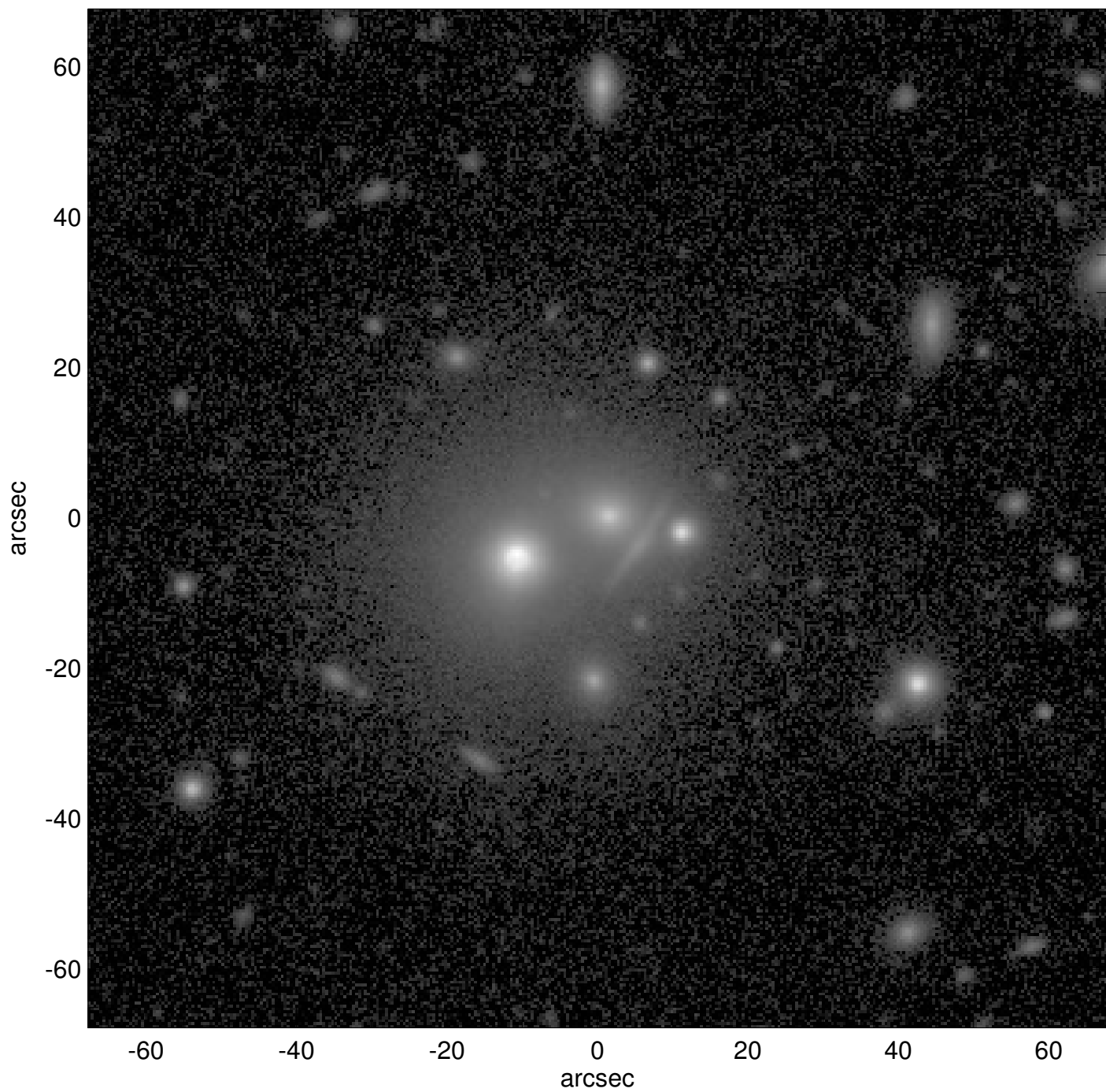
PGC1141939
