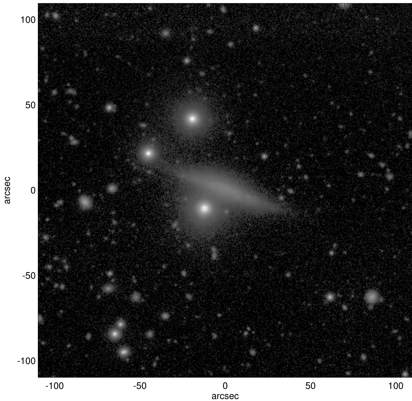
PGC1154022
