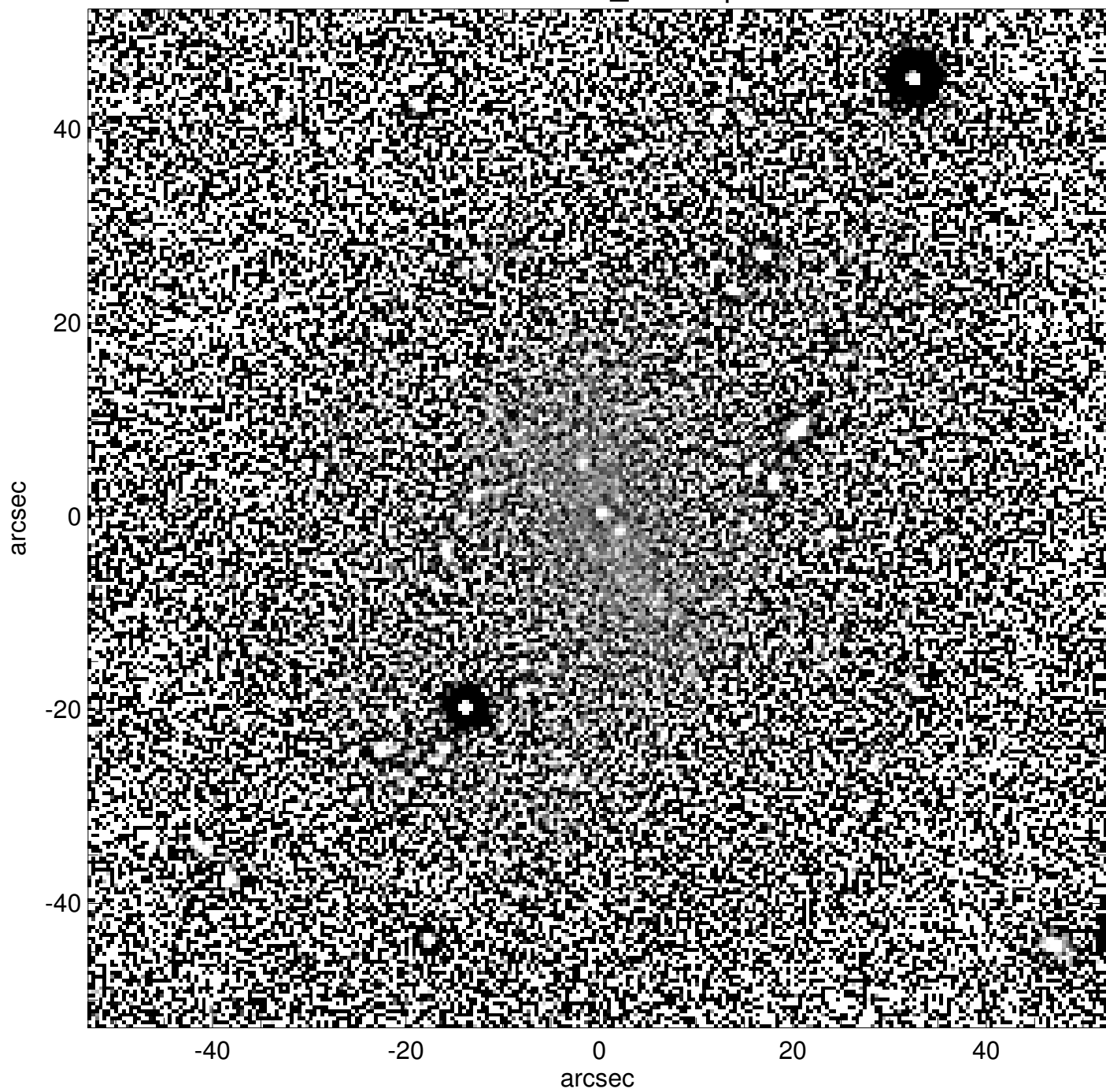
UGC00328_unsharp
