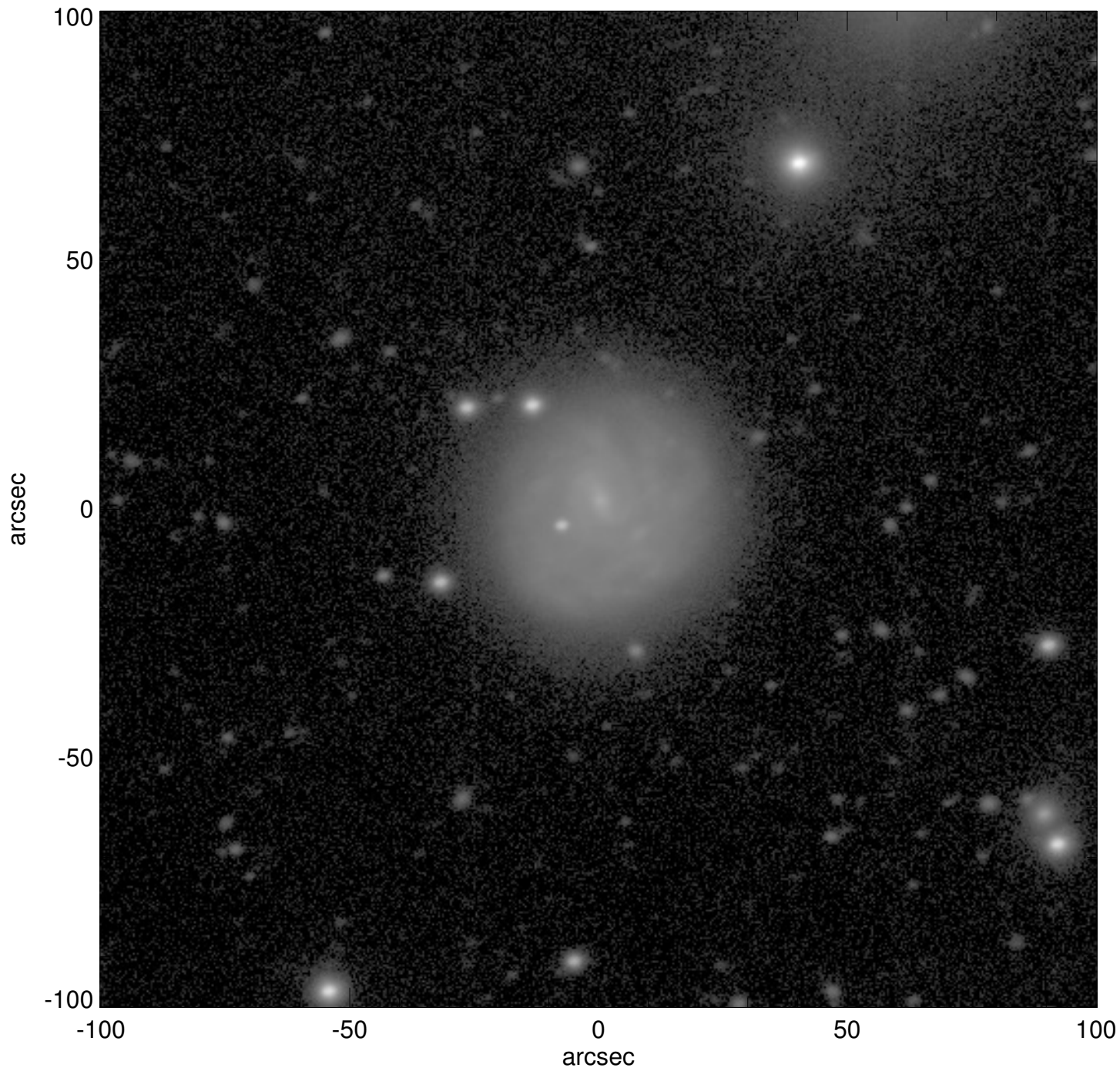
UGC00790
