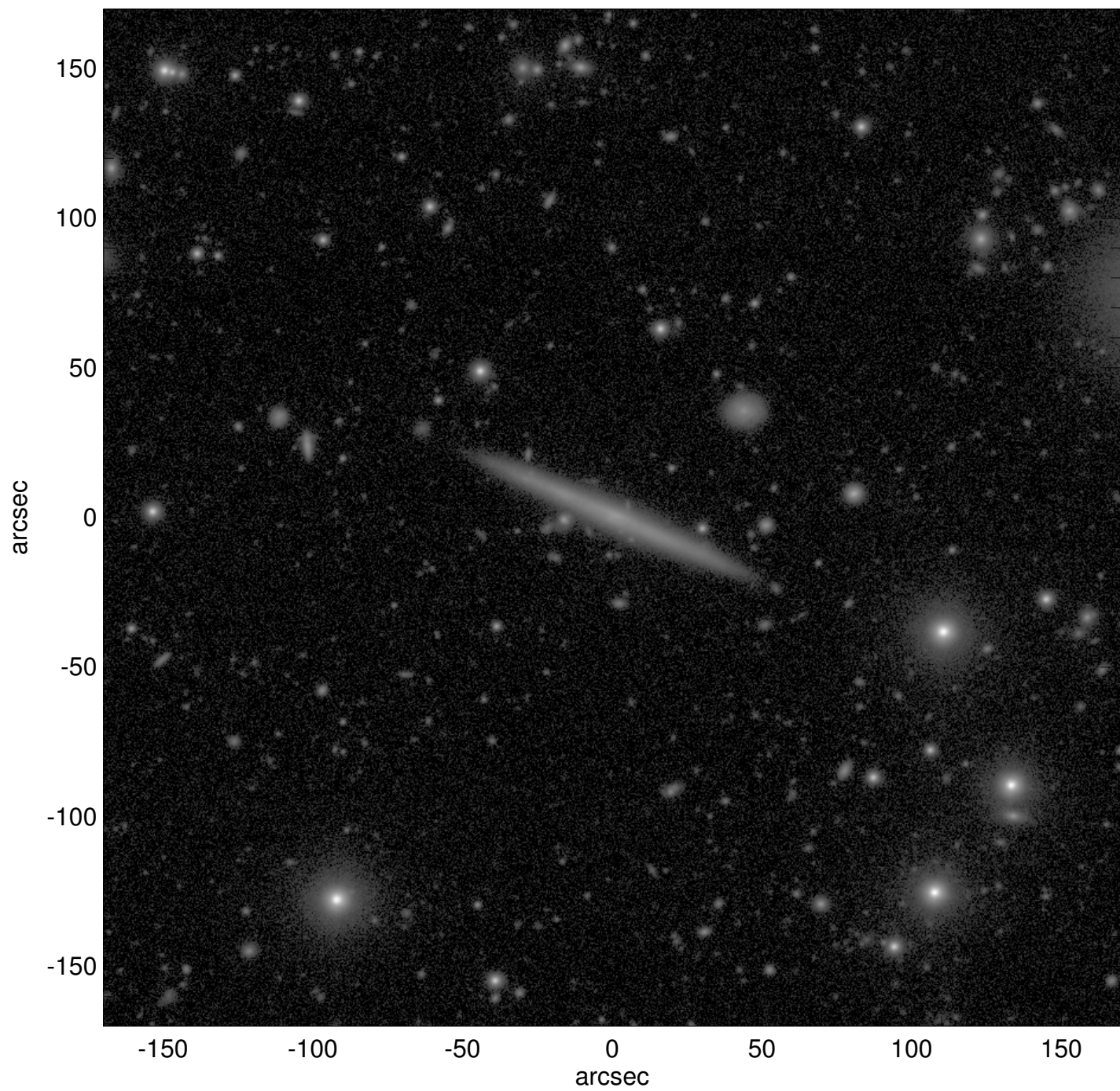
UGC00847
