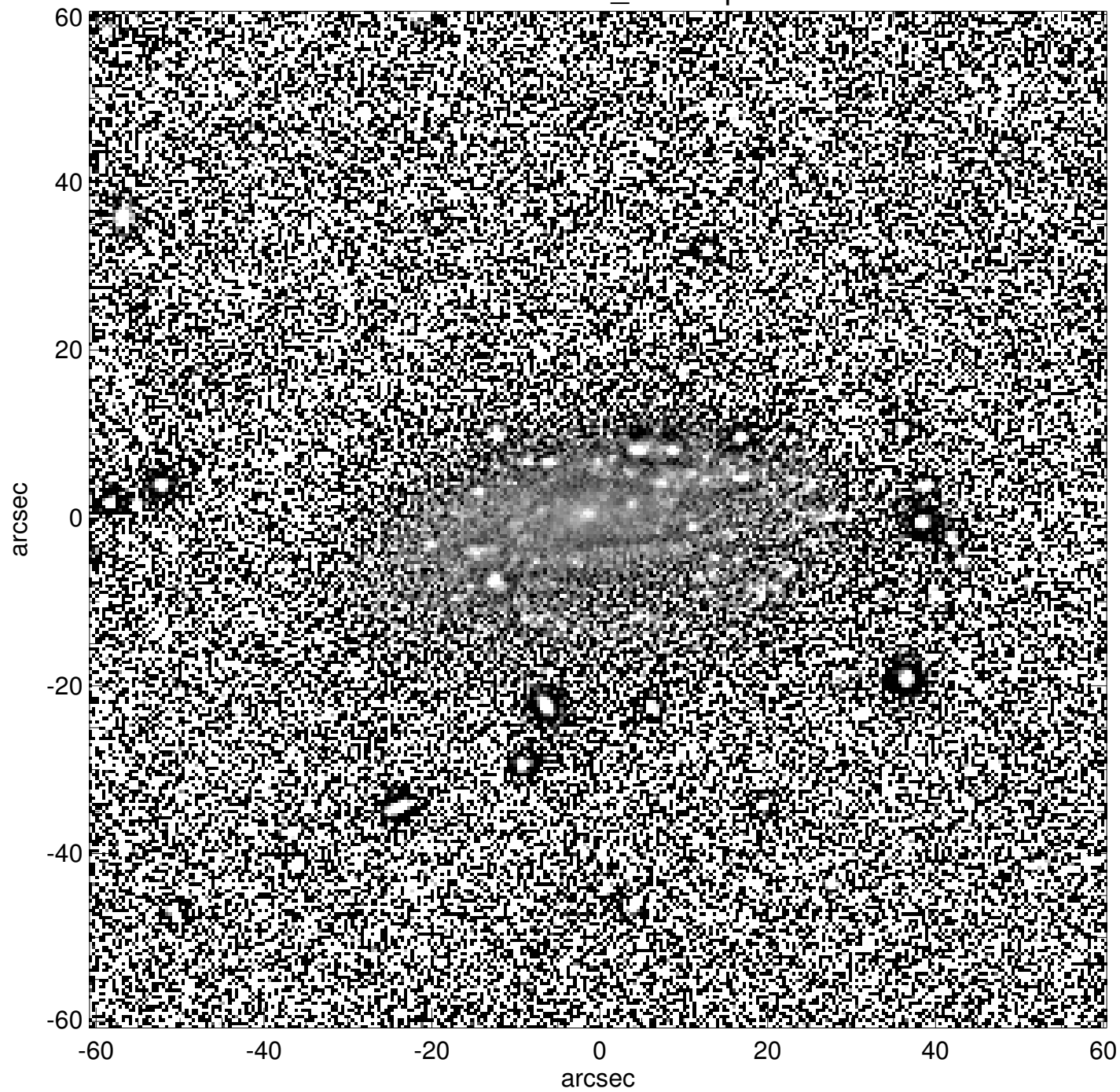
UGC00894_unsharp
