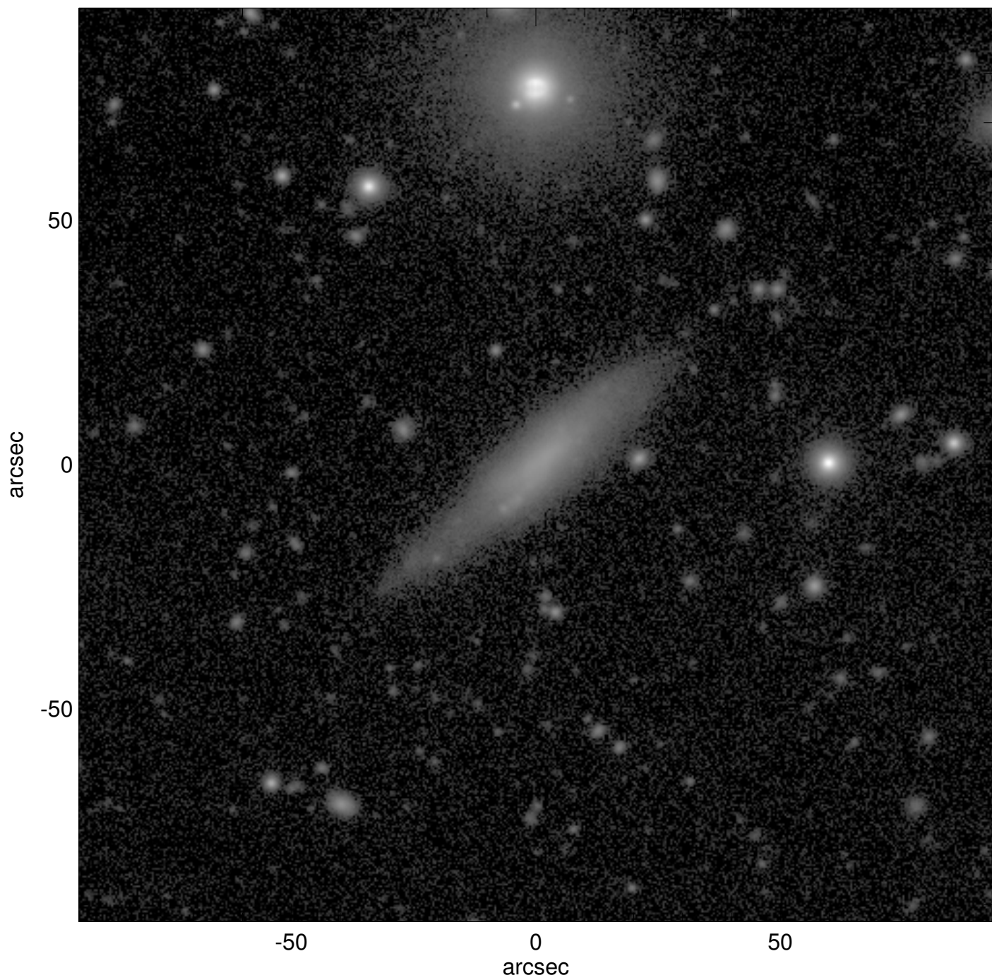
UGC00998
