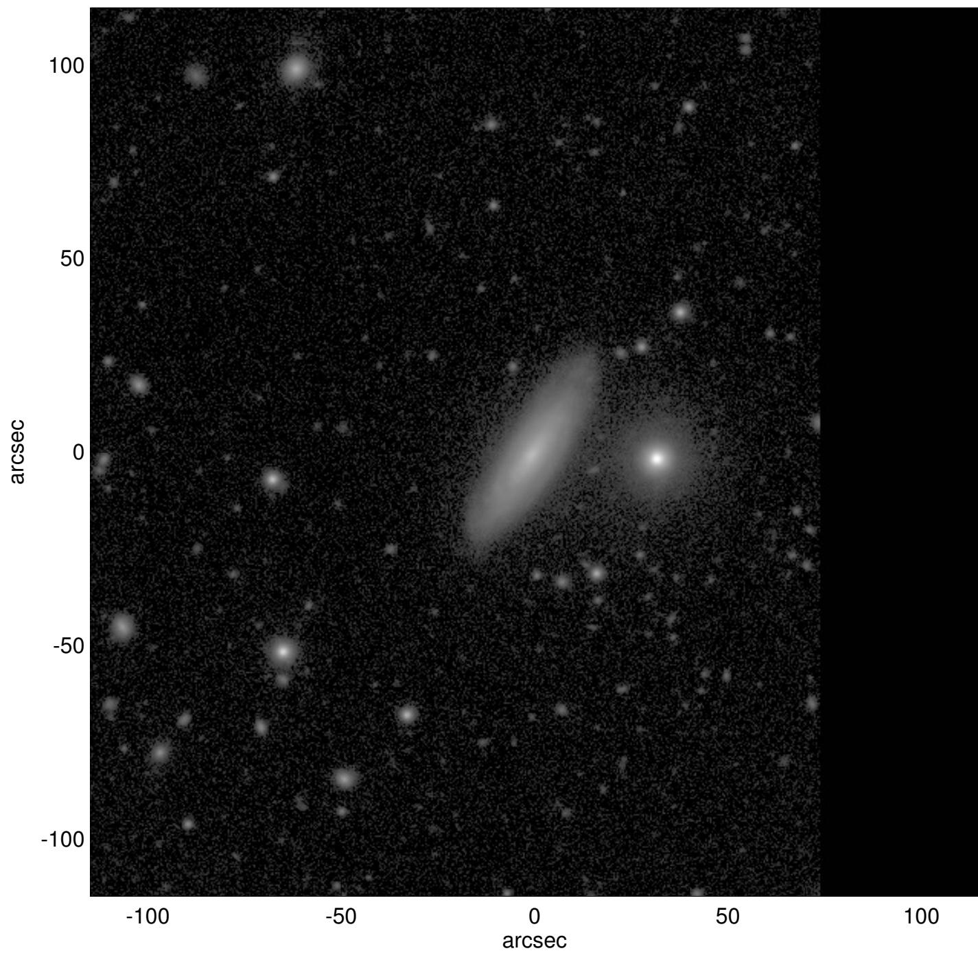
UGC01481
