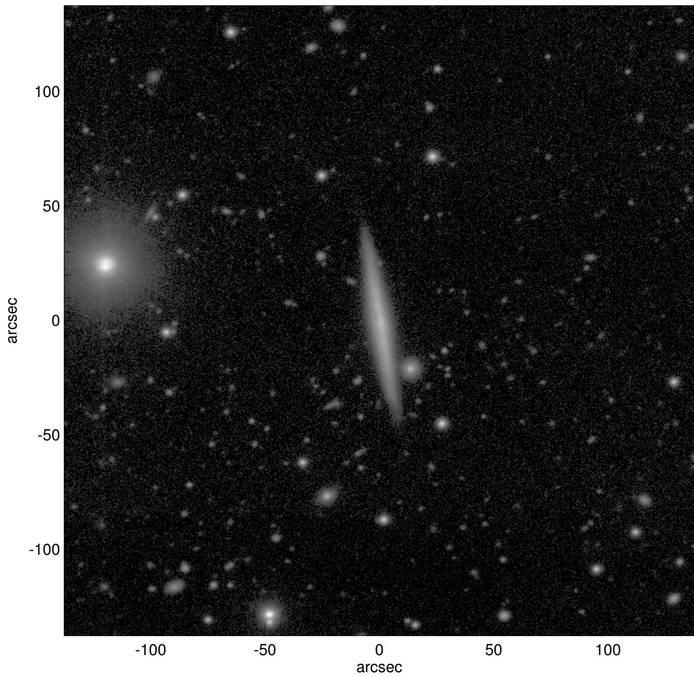
UGC02404
