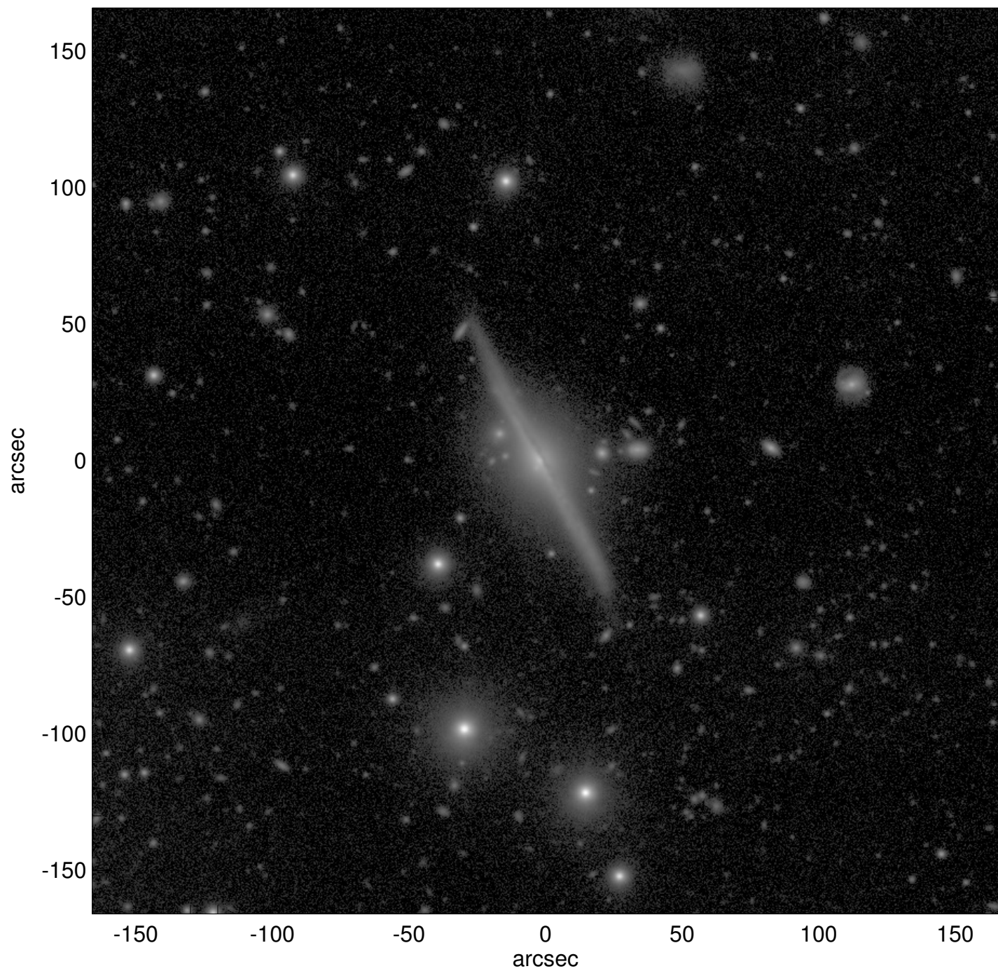
UGC02587
