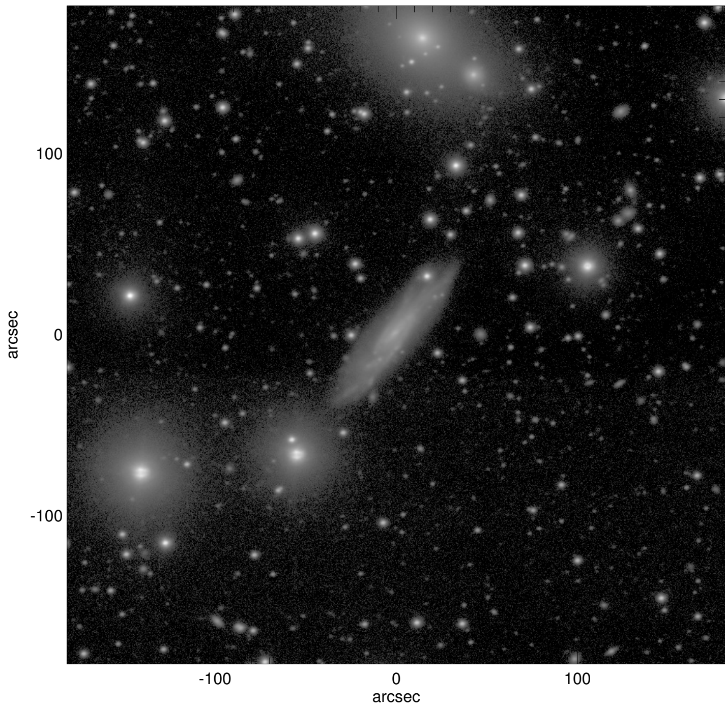
UGC11724
