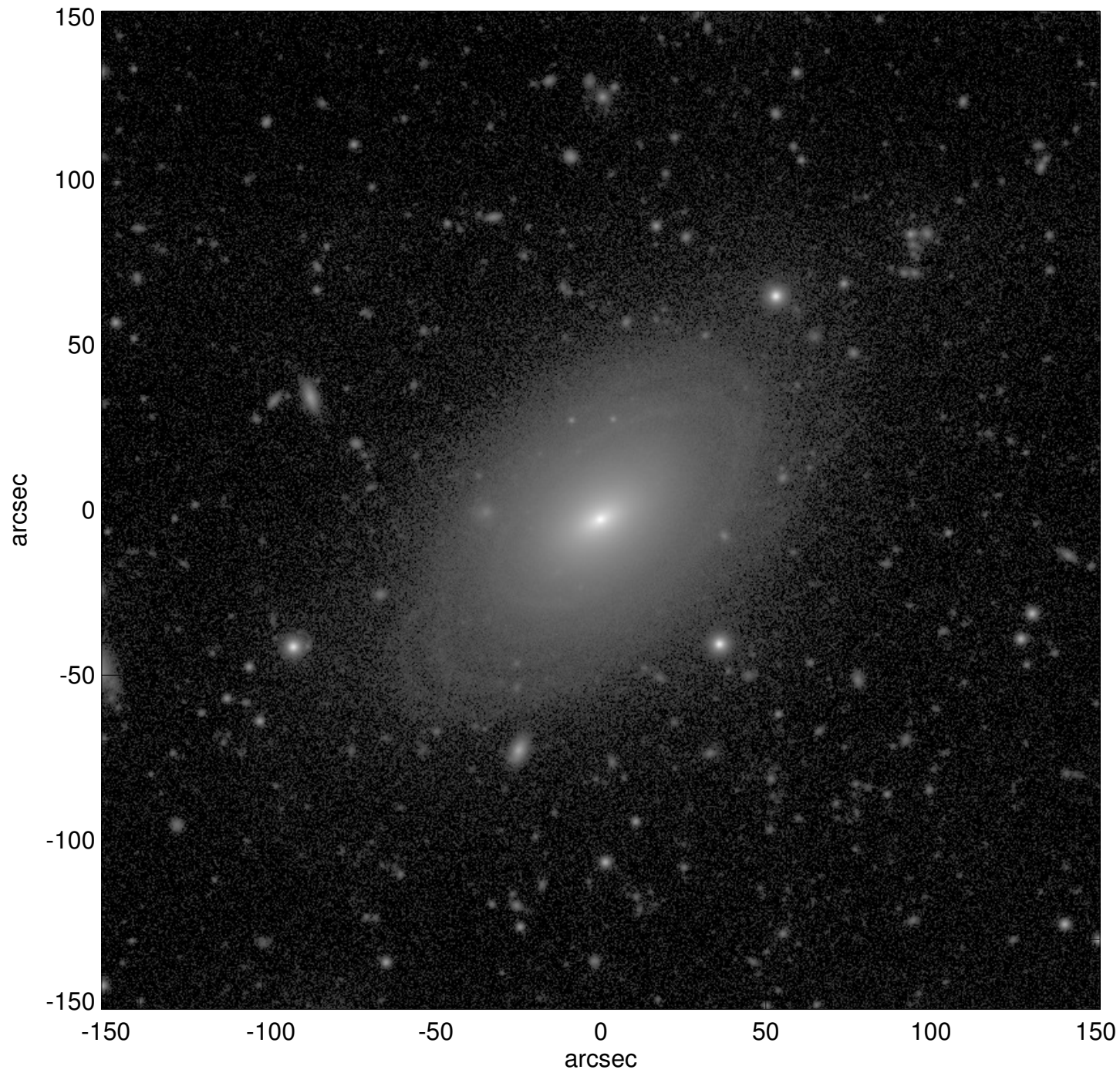
NGC0934
