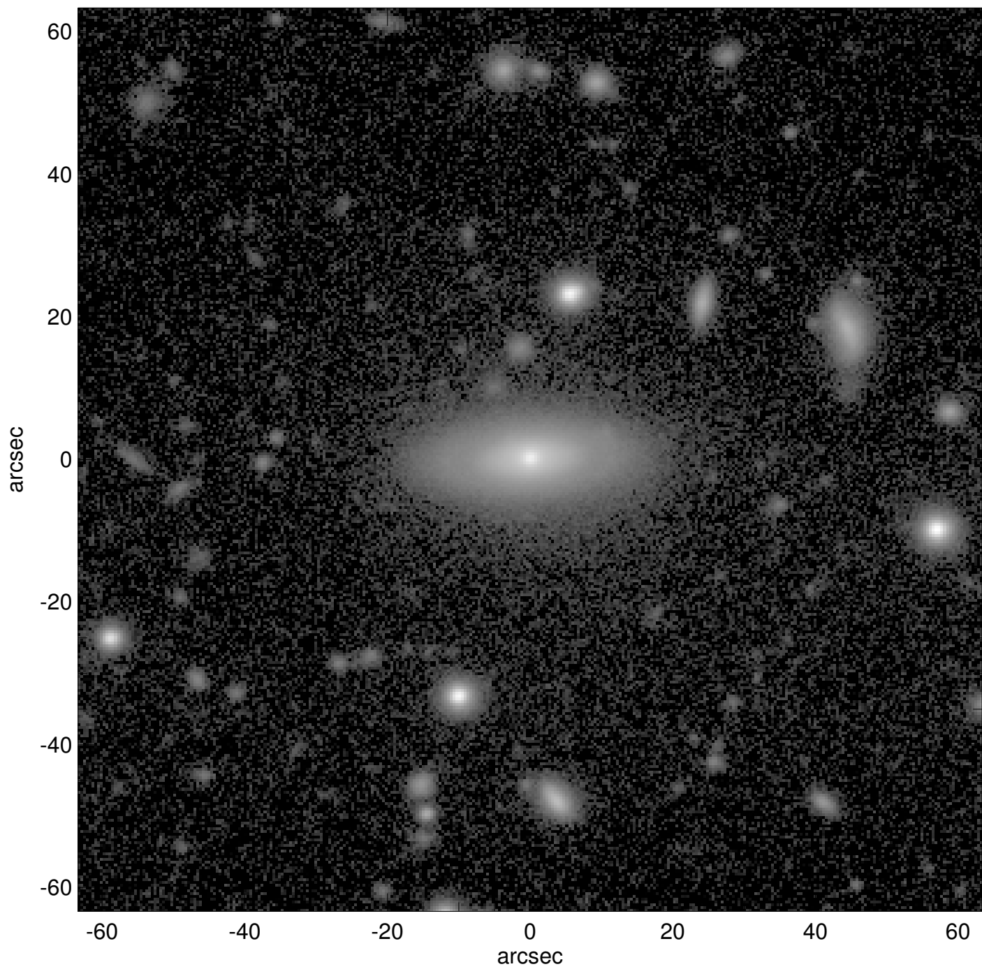
PGC1175423
