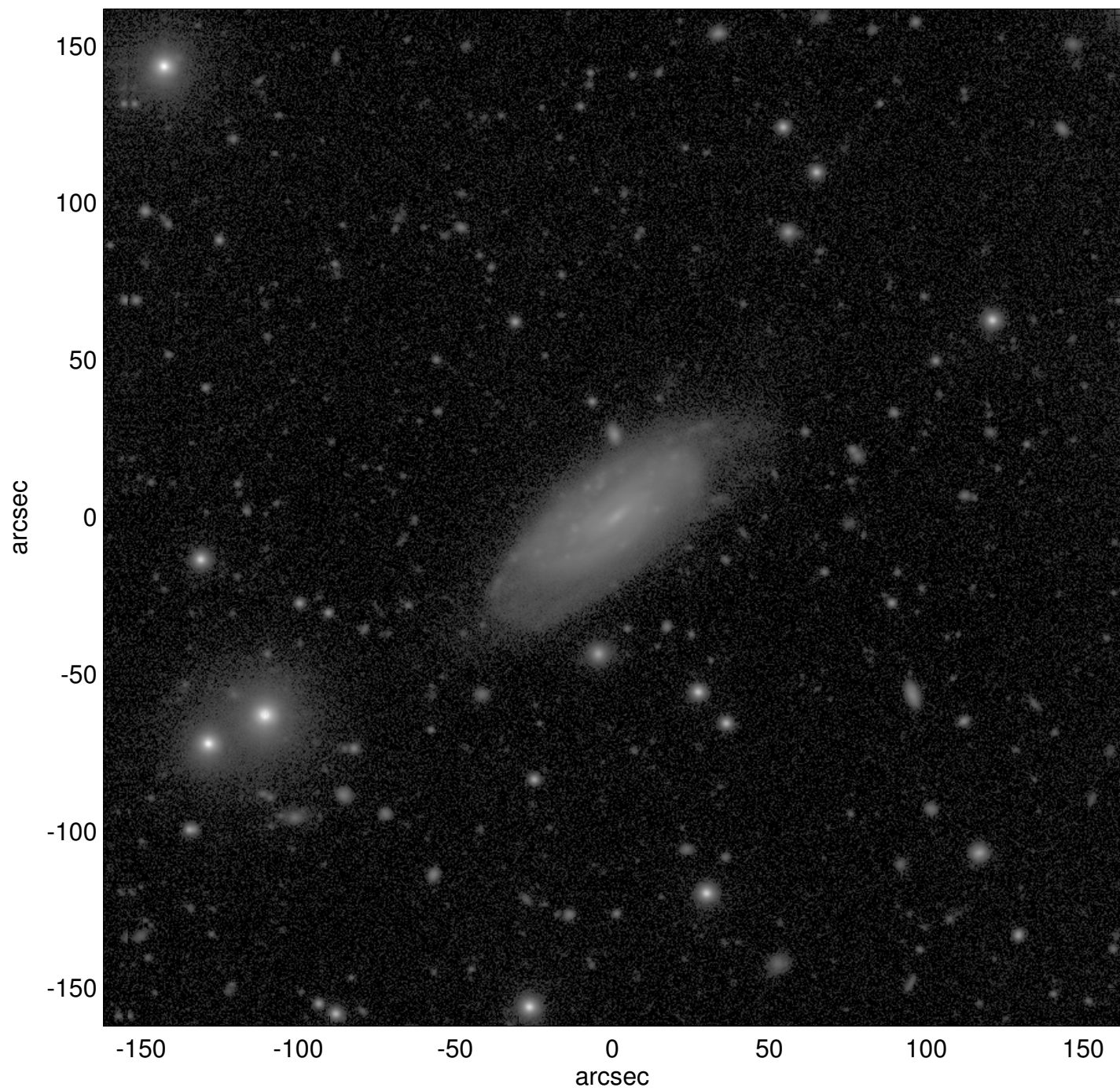
UGC00272
