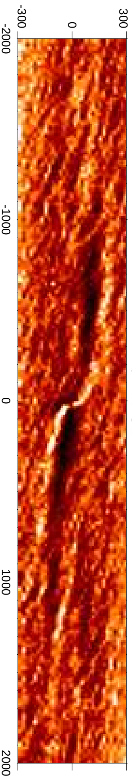
I/F IMAGE
